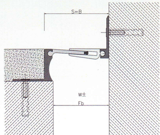
E 423/ALR-090 mit Dichtlippe / with sealing lip
