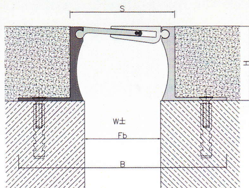
423/ALR-090 mit Dichtlippe / with sealing lip
